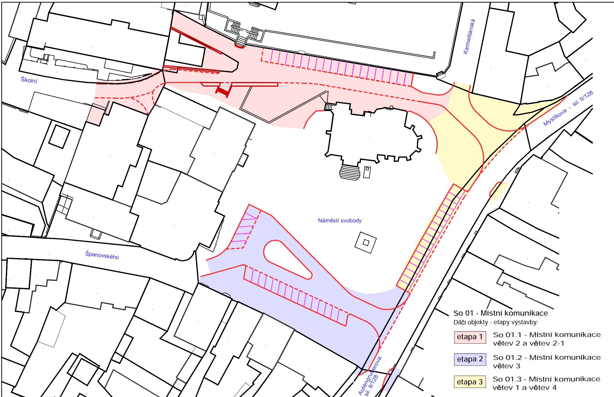
Pacov, náměstí Svobody - Stavební úpravy
